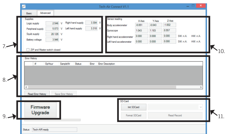
Figura 12 - Geavanceerd Scherm Tech-Air™ Aansluiting
