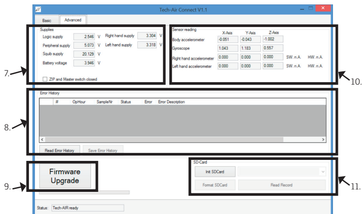
Figure 12 - Tech-Air™ Connect Erweiterter Bildschirm
