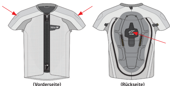
Abbildung 1 - Sensorpositionen.
