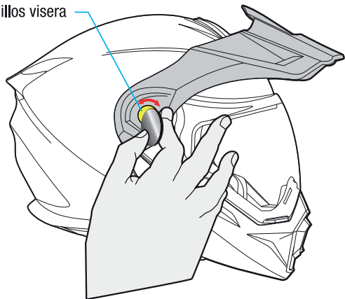
Tornillos visera
