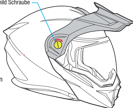
Helmschild Schraube
