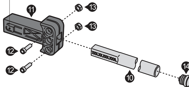
Lasche / Clip
