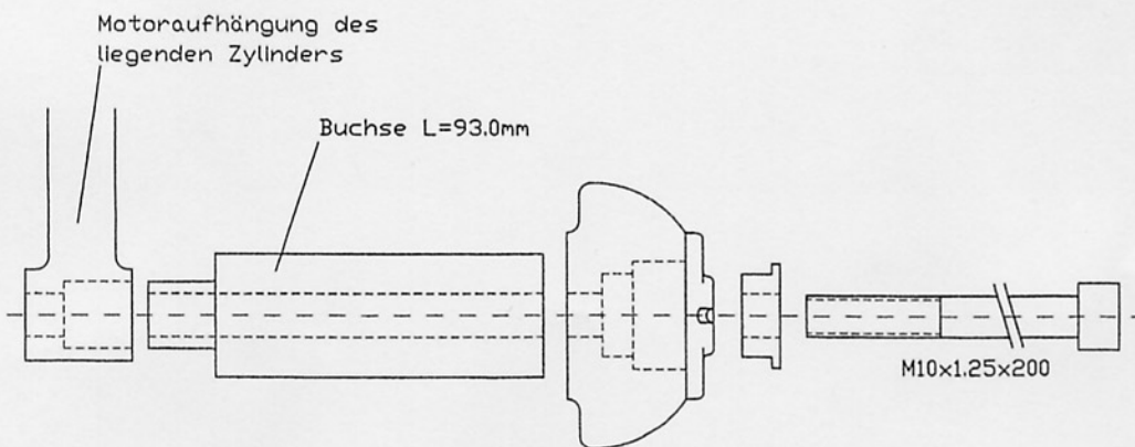
Montageteile links, Ansicht von vorn!
